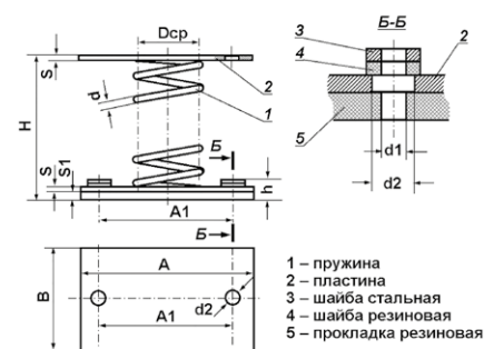
Схема 47. Виброизолятор
