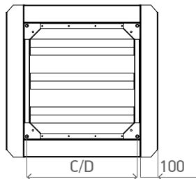
Табл. 7. Габаритные и присоединительные размеры монтажных стаканов /TSS_
