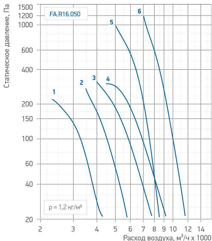
Табл. 20. Аэродинамические и акустические характеристики вентиляторов /FA.R16.050 (056)
