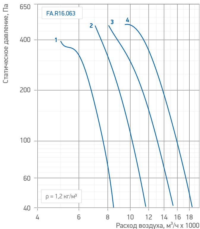
Гр. 12. Аэродинамические характеристики вентилятора / FA.R16.063
