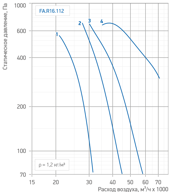
Табл. 23. Аэродинамические и акустические характеристики вентиляторов /FA.R16.100 (112)
