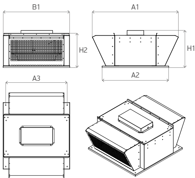
Табл. 2. Габаритно-весовые характеристики вентиляторов LM SAUGER /FB_
