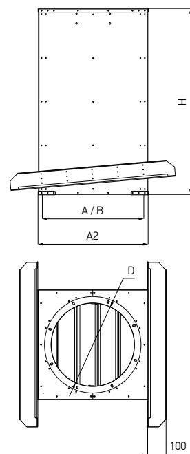
Схема 63. Станок монтажный с шумоглушителем и обратным клапаном для плоской кровли TSB.B_, TSD.B_, TSF.B_
