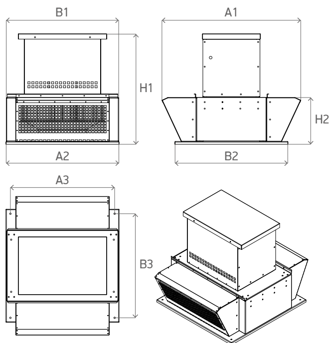
Схема 2. Габаритные характеристики вентиляторов /FPH
