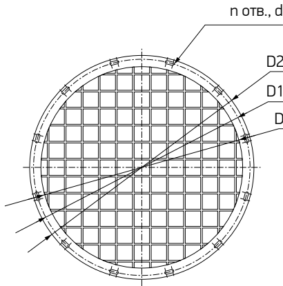
Схема 48. Защитная сетка
