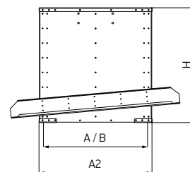
Схема 56. Станок монтажный с обратным клапаном приток для скатной кровли TSA.C_, TSC.C_, TSE.C_
