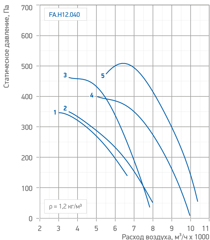
Табл. 26. Аэродинамические и акустические характеристики вентиляторов /FA.H12.040 (045)
