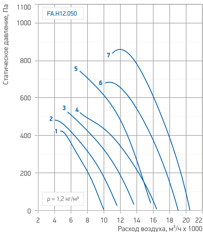
Табл. 27. Аэродинамические и акустические характеристики вентиляторов /FA.H12.050 (056)
