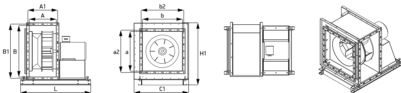
Схема 21. Габаритные и присоединительные характеристики вентиляторов LM PRO WURFEL FAN /FPR (выхлоп вправо)
