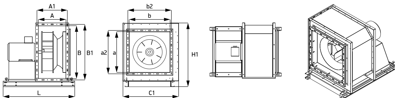
Схема 21. Габаритные и присоединительные характеристики вентиляторов LM PRO WURFEL FAN /FPR (выхлоп вправо)
