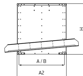
Схема 54. Стакан монтажный с обратным клапаном вытяжка для скатной кровли TSA.B_, TSC.B_, TSE.B_
