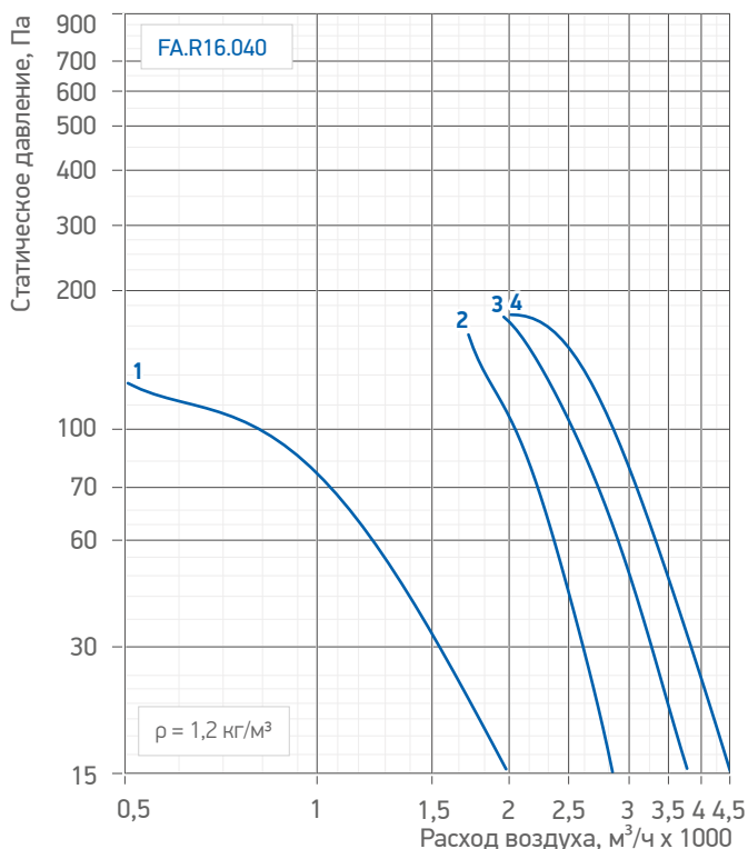
Гр. 8. Аэродинамические характеристики вентилятора /FA.R16.040
