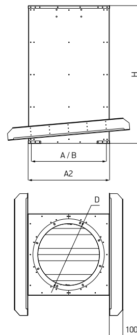
Схема 59. Станок монтажный с шумоглушителем для плоской кровли TSB.N_, TSD.N_, TSF.N_
