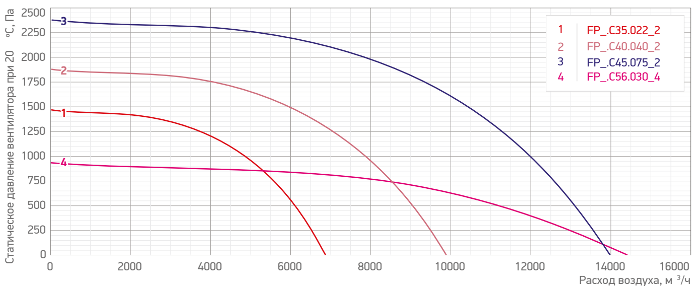
Табл. 11. Электрические характеристики вентиляторов LM PRO WURFEL FAN /FP_ (расход до 14 000 м³/ч)
