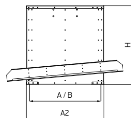
Схема 50. Стакан монтажный для скатной кровли TSA.N_, TSC.N_, TSE.N_
