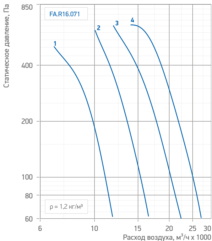
Гр. 13. Аэродинамические характеристики вентилятора / FA.R16.071
