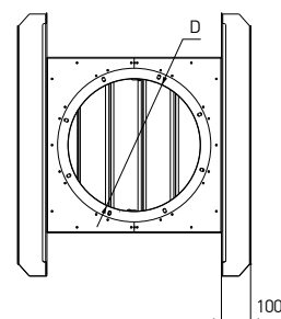
Схема 57. Станок монтажный с обратным клапаном приток для плоской кровли TSA.C_, TSC.C_, TSE.C_
