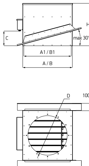
Схема 66. Иллюстрация исполнения стакана монтажного для скатной кровли кровли TSA.F2, TSE.F2, TSC.F2
