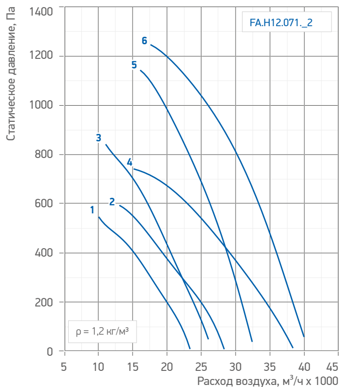
Гр. 26. Аэродинамические характеристики вентилятора / FA.H12.071._2
