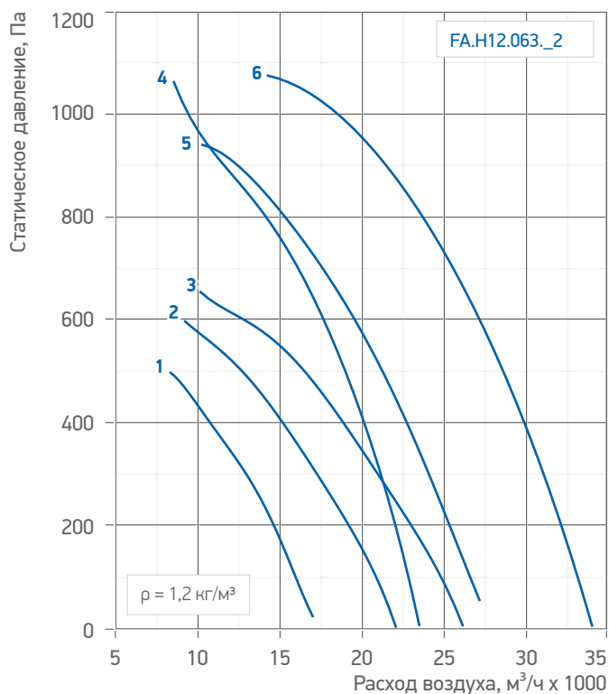
Гр. 24. Аэродинамические характеристики вентилятора / FA.H12.063_2
