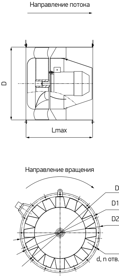
Схема 37. Исполнение F
