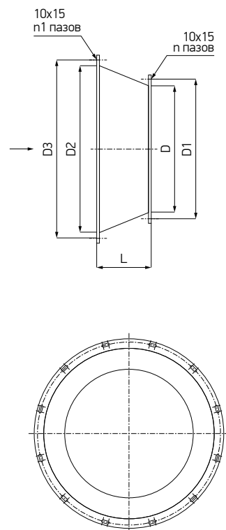
Схема 41. Конфузор на всасе
