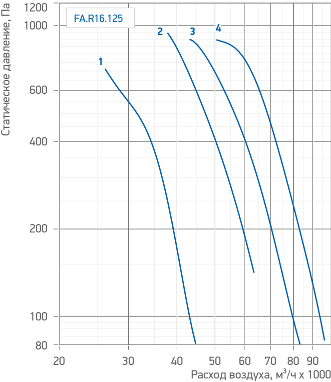
Табл. 24. Аэродинамические и акустические характеристики вентилятора /FA.R16.125
