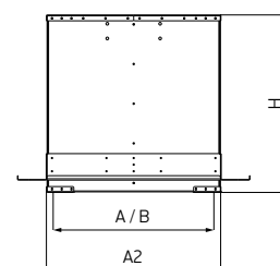
Схема 57. Станок монтажный с обратным клапаном приток для плоской кровли TSA.C_, TSC.C_, TSE.C_
