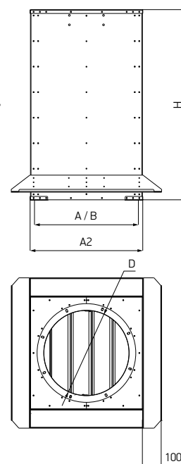
Схема 65. Станок монтажный с шумоглушителем и обратным клапаном для плоской кровли TSB.C_, TSD.C_, TSF.C_
