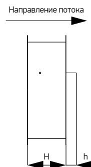
Схема 45. Клапан обратный вертикальный для работы на вытяжку VO.1, VOK.1, VOD.1
