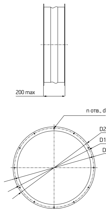
Схема 49. Гибкая вставка
