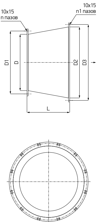
Схема 42. Диффузор на выхлопе
