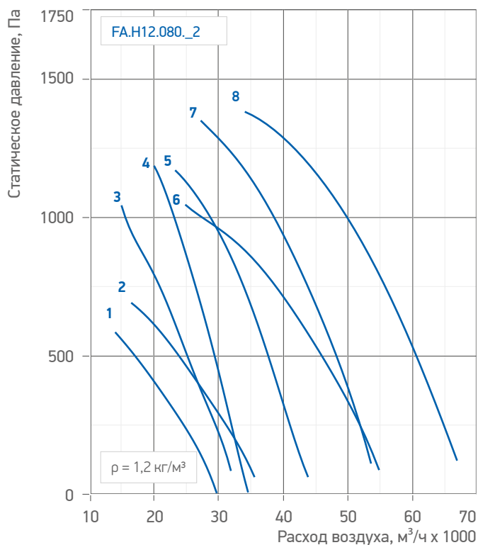
Гр. 28. Аэродинамические характеристики вентилятора / FA.H12.080._2
