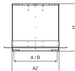
Схема 55. Стакан монтажный с обратным клапаном вытяжка для плоской кровли TSA.B_, TSC.B_, TSE.B_
