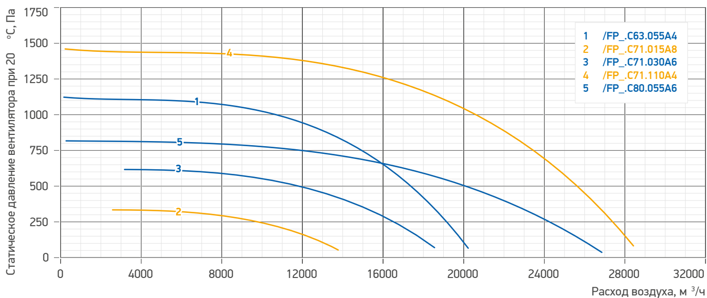
Гр. 3. Аэродинамические характеристики вентиляторов LM SAUGER /FP_ (продолжение)
