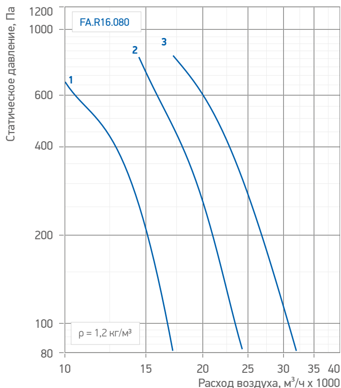
Табл. 22. Аэродинамические и акустические характеристики вентиляторов /FA.R16.080 (090)
