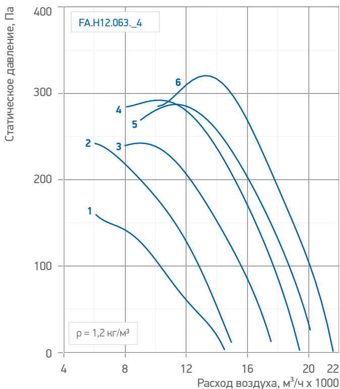
Гр. 23. Аэродинамические характеристики вентилятора / FA.H12.063_4
