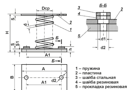
Схема 24. Виброизоляторы /DO
