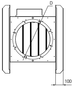
Схема 53. Стакан монтажный с клапаном для плоской кровли TSA.V_, TSC.V_, TSE.V_
