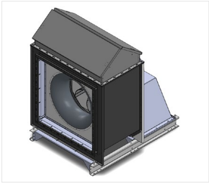
Рис. 8. Козырёк для вентилятора /Vf
