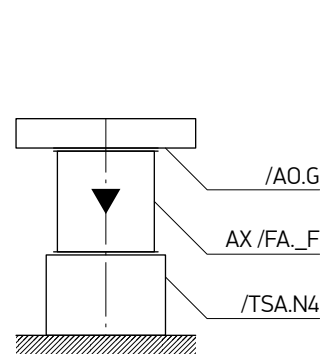
Схема 28. Пример исполнения 3
