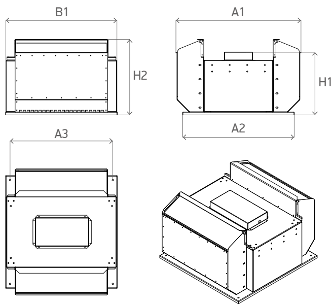
Схема 5. Габаритные характеристики вентиляторов /FBV
