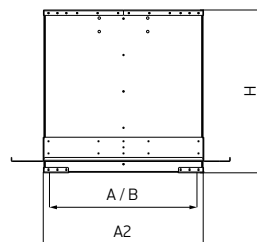
Схема 51. Стакан монтажный для плоской кровли TSA.N_, TSC.N_, TSE.N_
