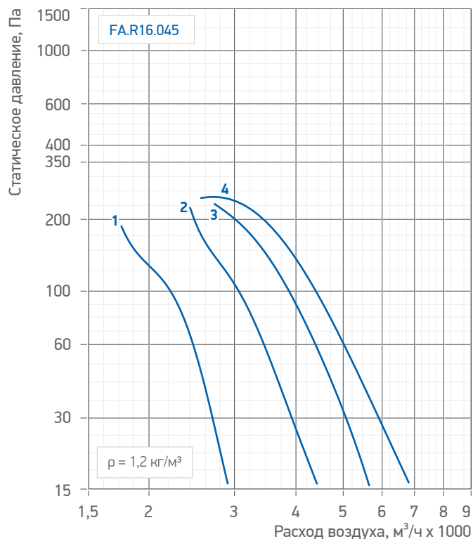
Гр. 9. Аэродинамические характеристики вентилятора /FA.R16.045
