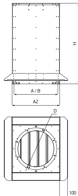
Схема 63. Станок монтажный с шумоглушителем и обратным клапаном для плоской кровли TSB.B_, TSD.B_, TSF.B_
