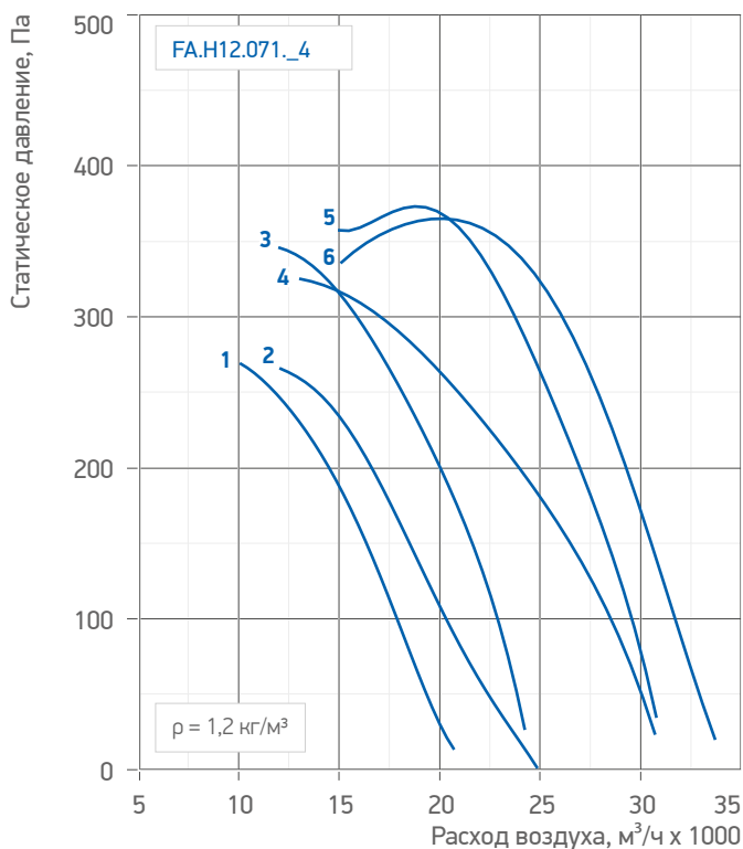
Гр. 25. Аэродинамические характеристики вентилятора / FA.H12.071._4
