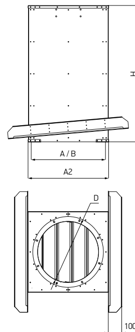
Схема 65. Станок монтажный с шумоглушителем и обратным клапаном для плоской кровли TSB.C_, TSD.C_, TSF.C_
