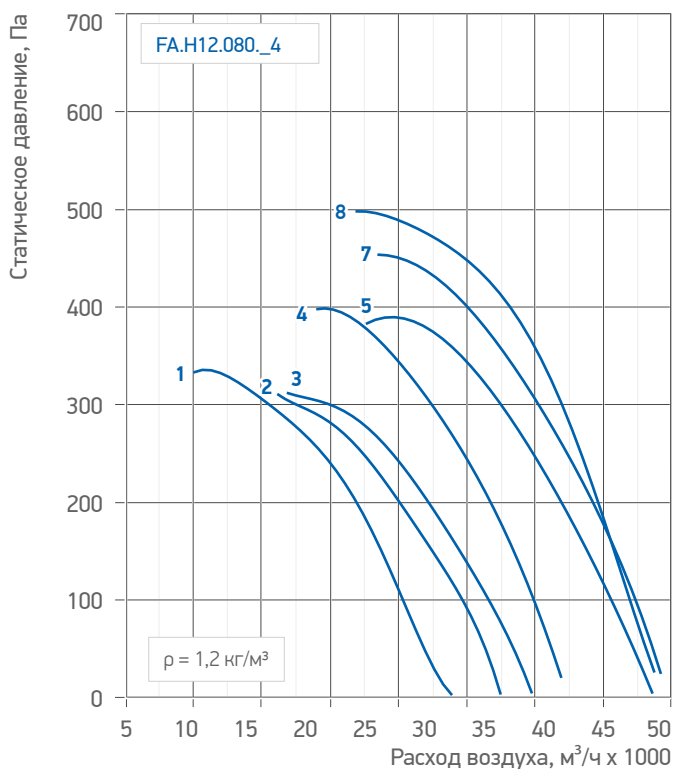
Табл. 30. Аэродинамические и акустические характеристики вентилятора /FA.H12.080
