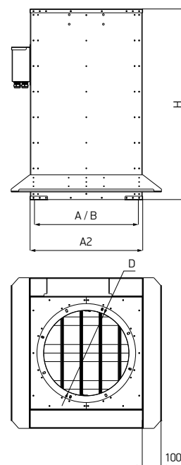
Схема 61. Станок монтажный с шумоглушителем и клапаном для плоской кровли TSB.V_, TSD.V_, TSF.V_
