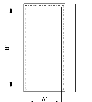
Схема 23. Гибкая вставка /G.G
