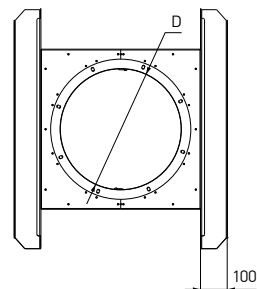
Схема 51. Стакан монтажный для плоской кровли TSA.N_, TSC.N_, TSE.N_
