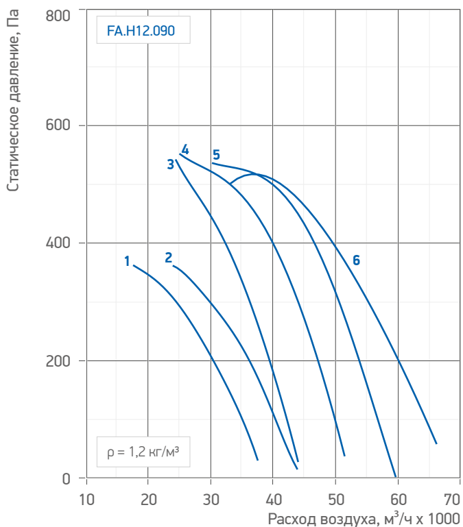
Табл. 31. Аэродинамические и акустические характеристики вентиляторов /FA.H12.090 (100_4)
