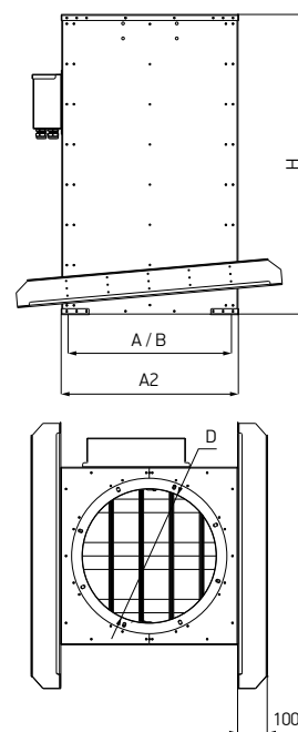
Схема 61. Станок монтажный с шумоглушителем и клапаном для плоской кровли TSB.V_, TSD.V_, TSF.V_
