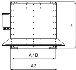
Схема 53. Стакан монтажный с клапаном для плоской кровли TSA.V_, TSC.V_, TSE.V_
