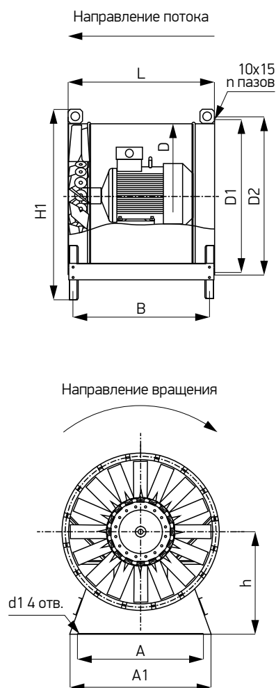
Схема 40. Исполнение S
