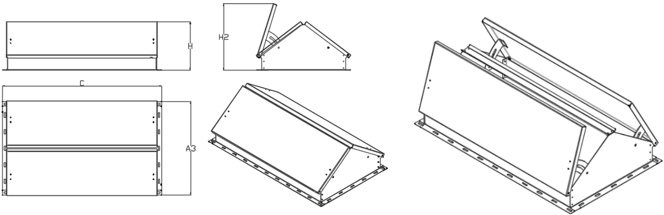
Схема 25. Габаритные характеристики козырька для вентилятора /Vf
