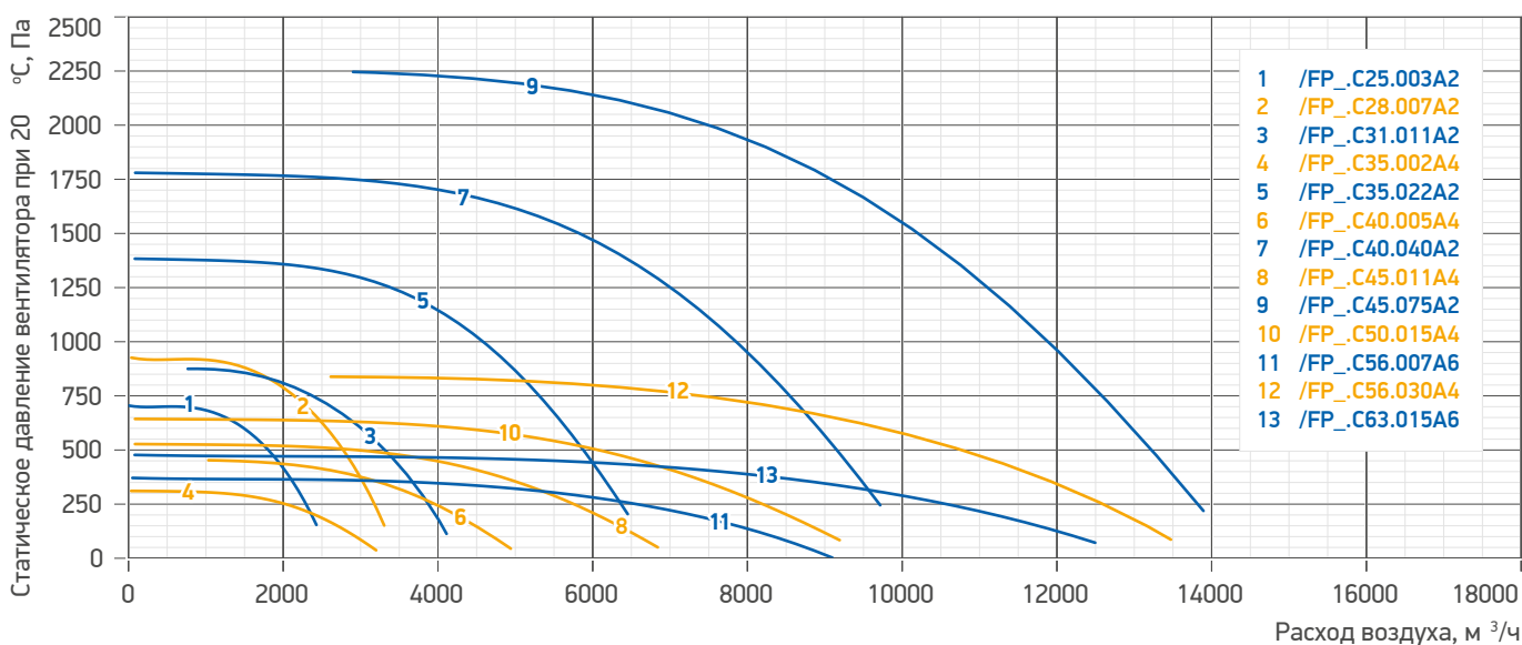
Гр. 1. Аэродинамические характеристики вентиляторов LM SAUGER /FP_
