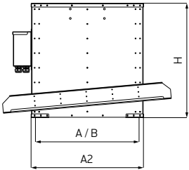
Схема 52. Стакан монтажный с клапаном для скатной кровли TSA.V_, TSC.V_, TSE.V_
