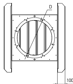
Схема 55. Стакан монтажный с обратным клапаном вытяжка для плоской кровли TSA.B_, TSC.B_, TSE.B_
