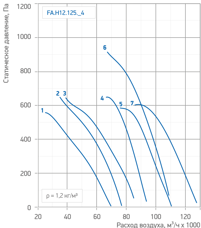
Табл. 33. Аэродинамические и акустические характеристики вентиляторов /FA.H12.112_6 (125_4)
