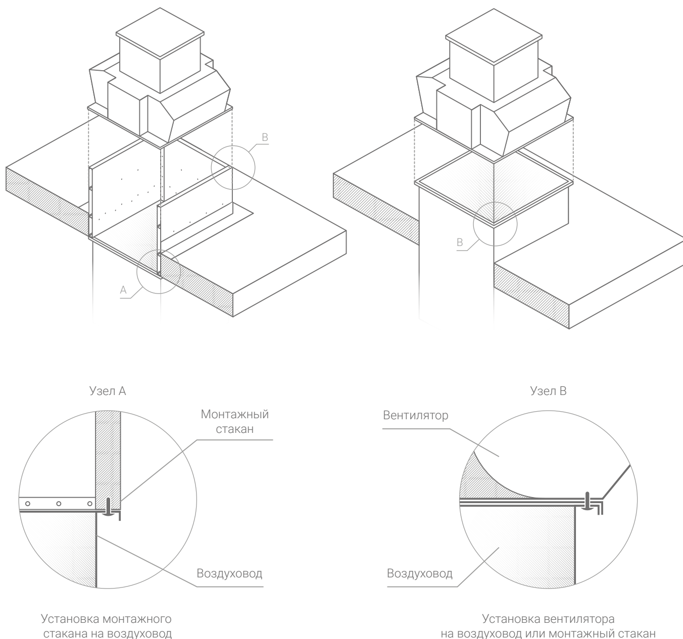
Схема 1. Узел крепления монтажного стакана к воздуховоду, вентилятора к монтажному стакану
