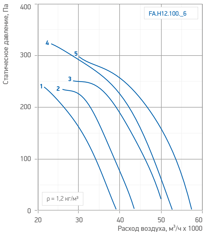
Табл. 32. Аэродинамические и акустические характеристики вентиляторов /FA.H12.100_6 (112_4)
