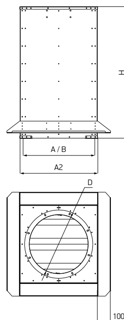
Схема 59. Станок монтажный с шумоглушителем для плоской кровли TSB.N_, TSD.N_, TSF.N_
