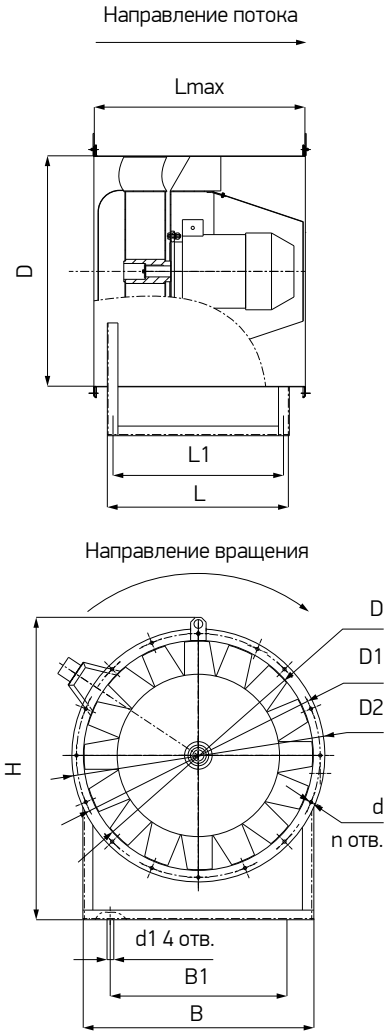
Схема 38. Исполнение S
