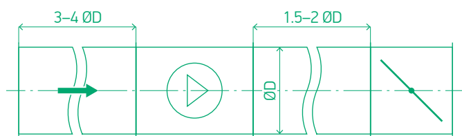
Схема 29. Монтаж в воздуховодах с элементами регулирования потока
