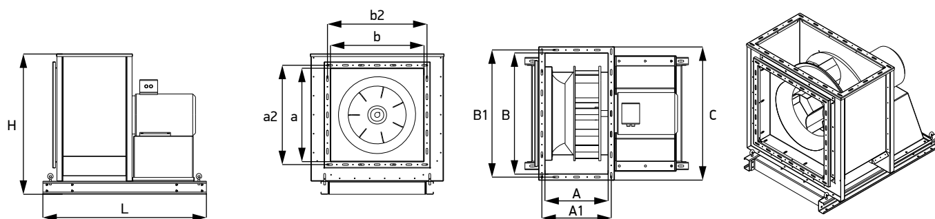
Схема 20. Габаритные и присоединительные характеристики вентиляторов LM PRO WURFEL FAN /FPL (выхлоп влево)
